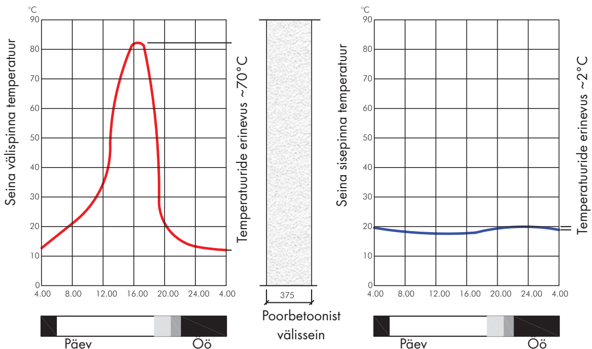
Graafik 2.4. AEROC välisseina soojusinerts
