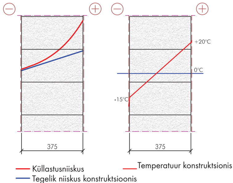
Graafik 2.3. AEROC EcoTerm Plus plokkidest viimistletud (väljas krohv ja sees pahtel) välisseina temperatuuri ja niiskuse graafikud
