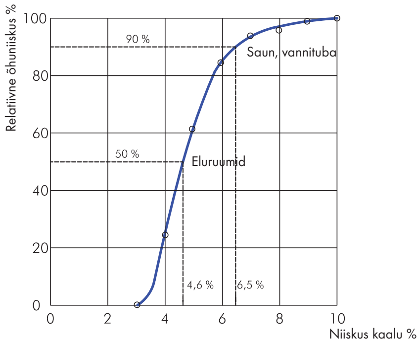
Graafik 2.2. Poorbetoonseinte tasakaaluniiskus sõltuvalt ruumide õhu relatiivsest niiskusest.
